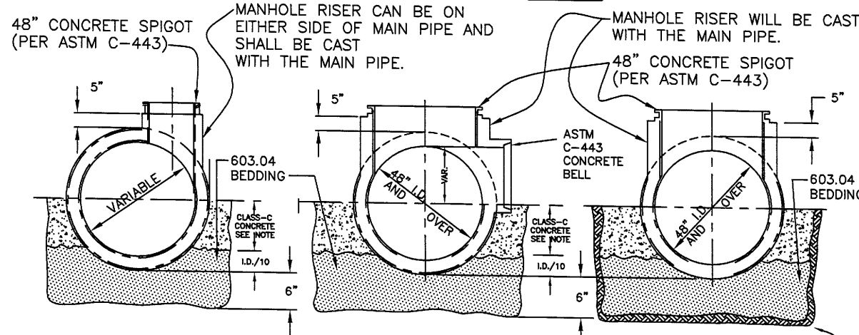
SECTION A-A PRECAST MANHOLE TEE WITH OFFSET MANHOLE RISER
